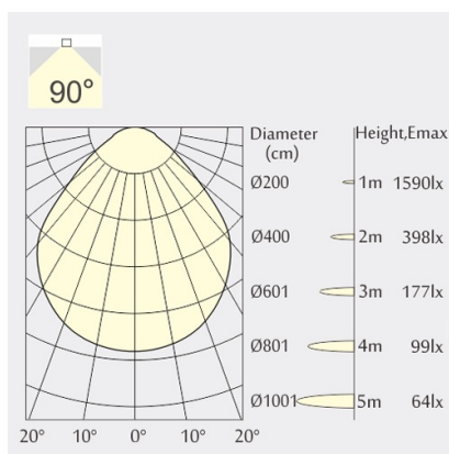
26W 4000K Ø600 mm
